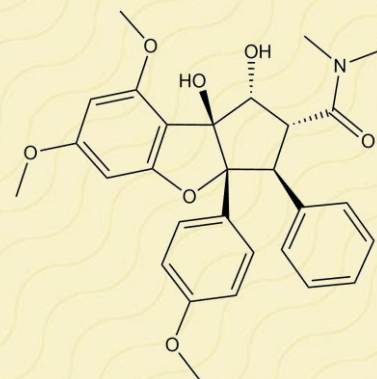
Rocaglamide
