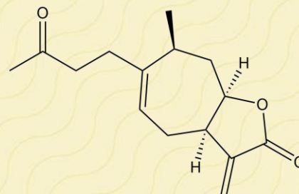
Tomentosin
