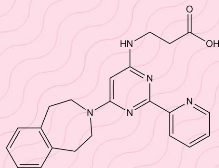
GSK J1
