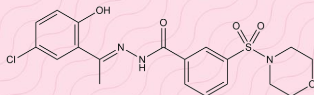
SP2509
