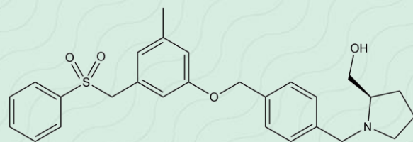
PF-543-HCl
