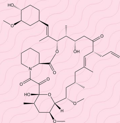
FK-506
